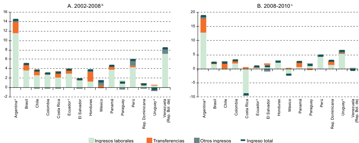
Gráfico I.5 AMÉRICA LATINA (15 PAÍSES): VARIACIÓN ANUAL DEL INGRESO TOTAL POR PERSONA Y DE CADA FUENTE EN LOS HOGARES POBRES a , 2002-2008 Y 2008-2010 (En porcentajes)
