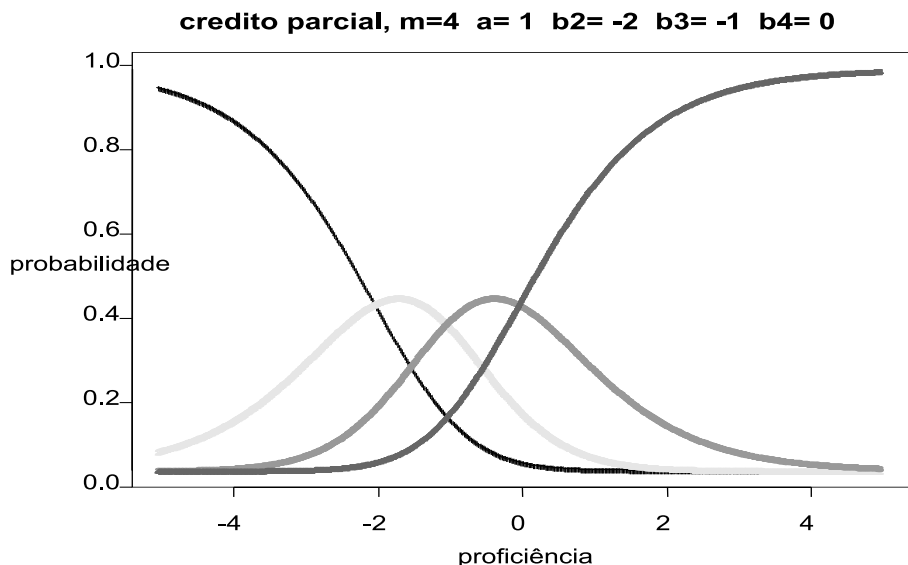
Figura 1: Curvas características de um modelo de crédito parcial com 4 graduações. Fonte: Bock e Muraki (2003).
