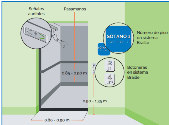
Figura 19: Elementos de un ascensor accesible
