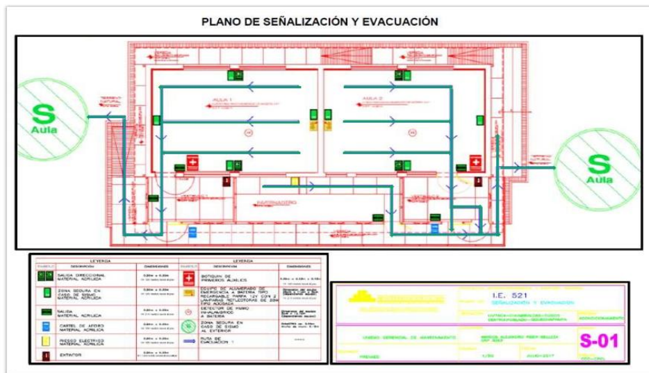
Figura 38: Plano de señalización y rutas de evacuación
