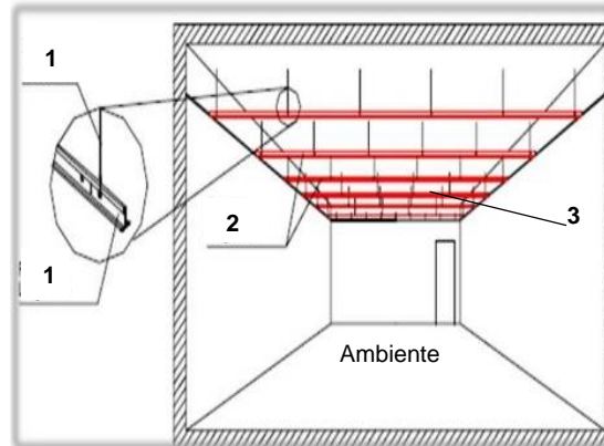
Figura N° 1-Esquema de falso cielorraso
